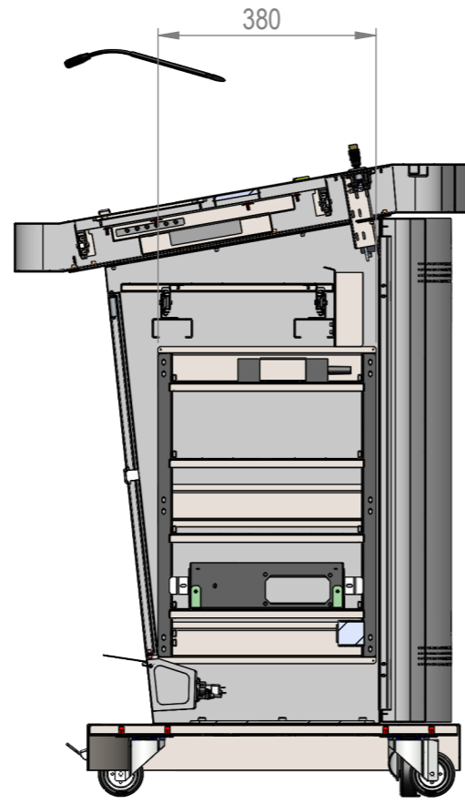
KESİT B-B ÖLÇEK 1 : 12
